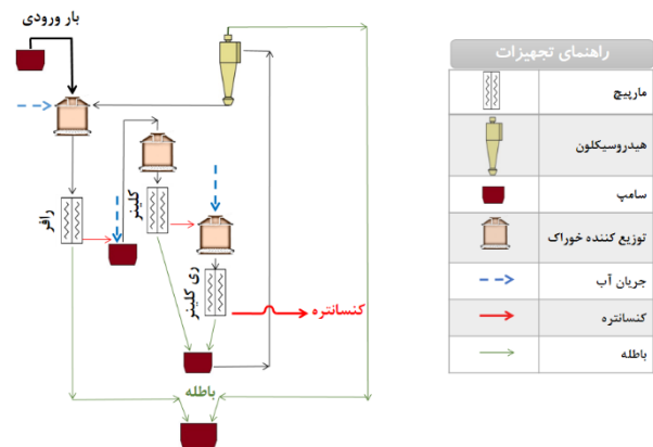
شکل ۱: مدار جداکننده‌های مارپیچی خط فرآوری باطله‌های خشک گل‌گهر
