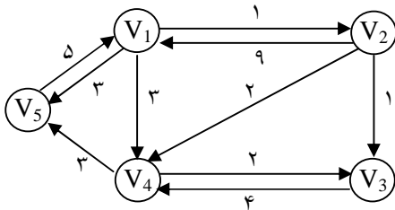
شکل ۳: نمونه‌ای از گراف جهت دار و وزن دار
