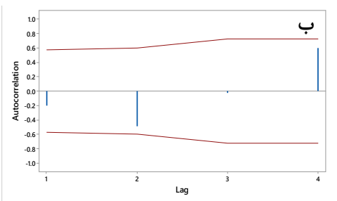
شکل ۲ - الف) نمودار پراکندگی برای داده‌های خرابی زیرسیستم هیدرولیک، ب) نمودار خودهمبستگی نما برای داده‌های خرابی زیرسیستم هیدرولیک
