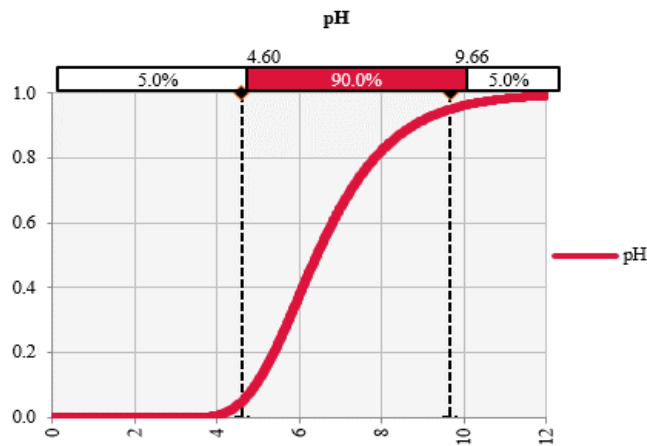
شکل ۹- نمودار تجمعی pH انباشتگاه باطله‌های زغالی البرز مرکزی حاصل از شبیه‌سازی.
