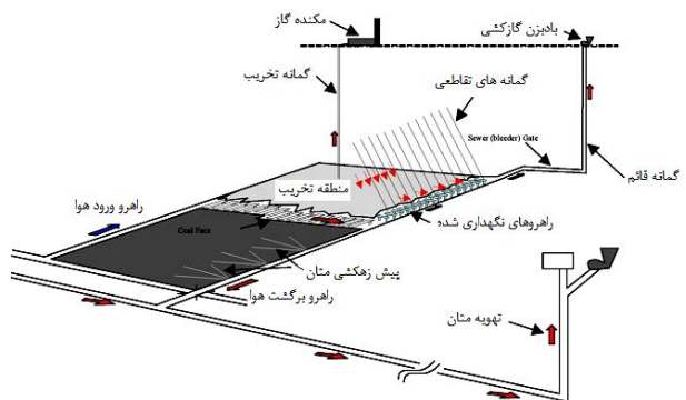
شکل ۱- شمایی از روش متان‌زدایی جبهه‌کار بلند [۵].
