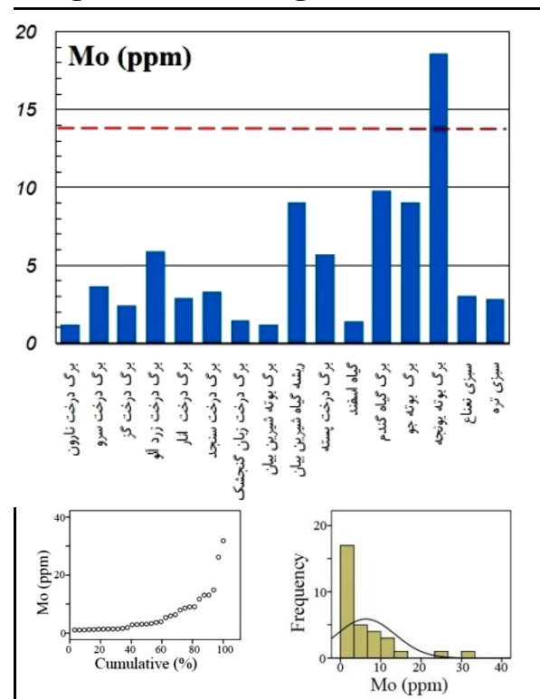
شکل ۳: نمودار توزیع، فراوانی و درصد تجمعی مولیبدن، خط چین میانگین جهانی عنصر در خاکستر گیاه [۳۷].
