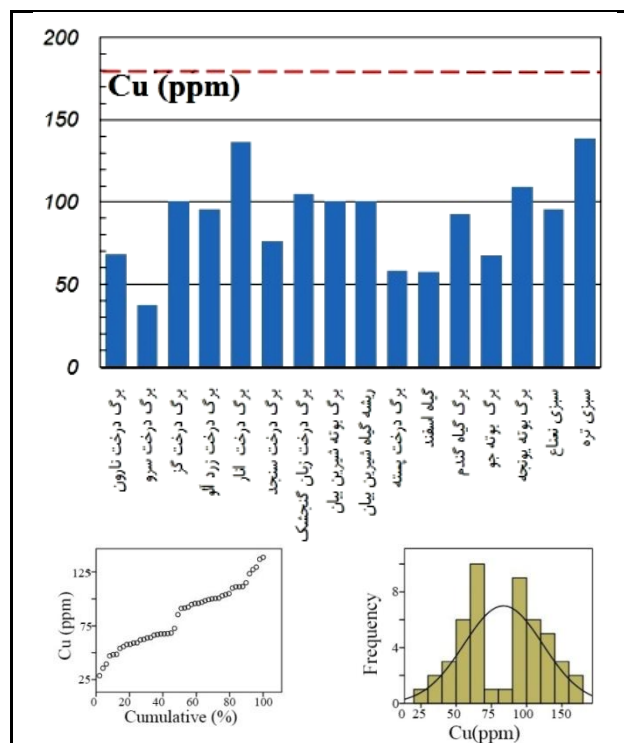
شکل ۲: نمودار توزیع، فراوانی و درصد تجمعی مس، خط چین میانگین جهانی عنصر در خاکستر گیاه [۳۷].
