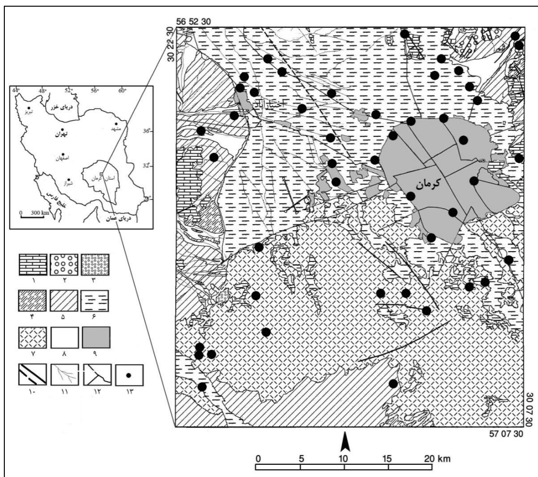
شکل ۱: نقشه زمین‌شناسی محدوده مورد مطالعه (۱- سنگ آهک های کرتاسه بالایی، ۲- کنگلومرای قاعده ایی پالتوسن، ۳- کنگلومرای نئوژن، ۴- پادگانه ها و نهشته‌های آبرفتی، ۵- آبرفت‌های جوان، ۶- پهنه های سیلتی -رسی، ۷- تپه‌های ماسه‌ای، ۸- آبرفت‌های عهد حاضر، ۹- مناطق مسکونی، ۱۰- گسل، ۱۱- آبراهه، ۱۲- خیابان و جاده، ۱۳- محل نمونه برداری (نقل با تغییرات از: [۳۹-۴۴]).
