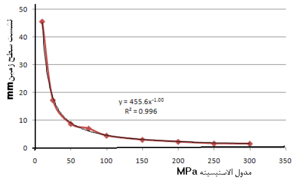
شکل ۱۶: رابطه نشست سطح زمین با مدول الاستیسیته
