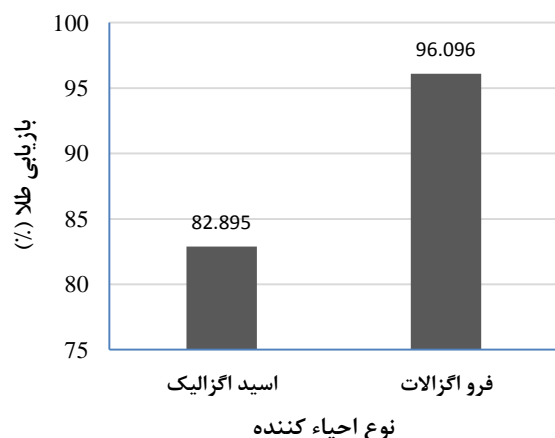
شکل ۲: مقایسه ترسیب طلا توسط اسید اگزالییک و فرو اگزالات (دما: ۸۰°C، pH=۶، زمان = ۶۰ min، غلظت فرو اگزالات ۵ g/l)
