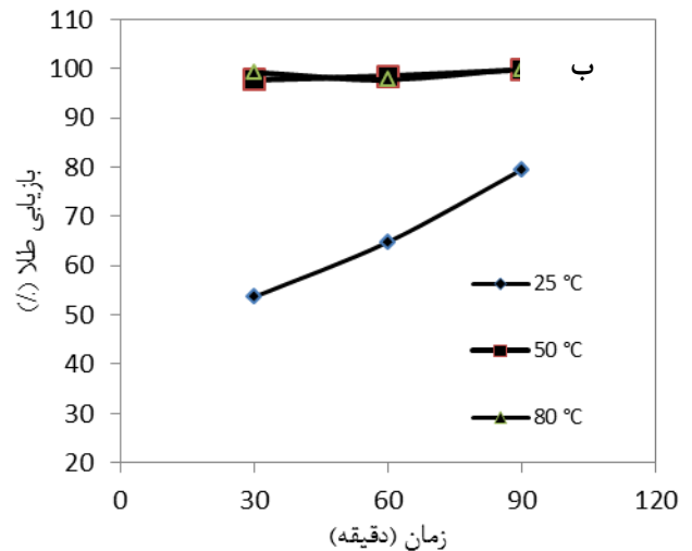
شکل ۷: تأثیر زمان بر بازیابی طلا از فاز آبی کلریدی با استفاده از فرو اگزالات (pH=۶، غلظت احیاء کننده: الف: ۵ g/l، ب: ۰.۵ g/l)
