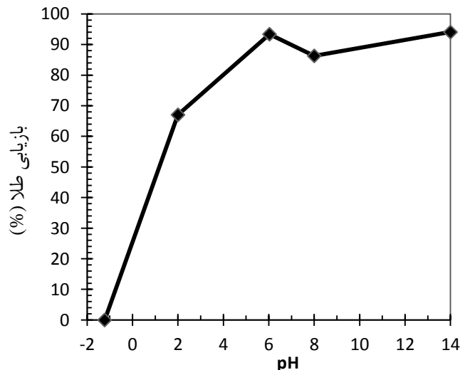
شکل ۶: تأثیر تغییرات pH بر بازیابی طلا از فاز آبی کلریدی با استفاده از فرو اگزالات (دما: 80^\circ\text{C} ، غلظت فرو اگزالات 5\text{ g/l} )
