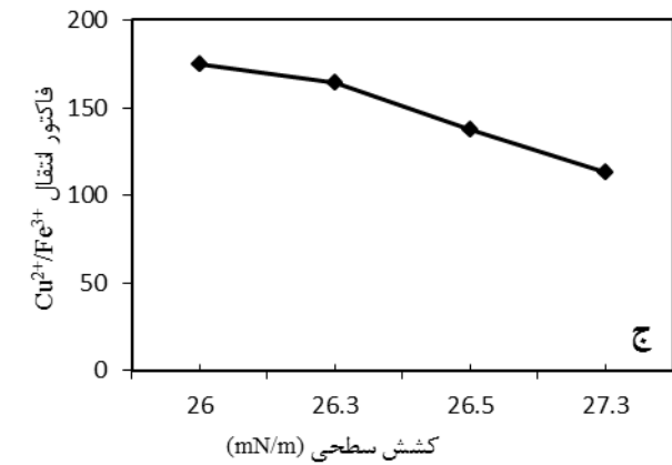
شکل ۵: تأثیر کشش سطحی رقیق کننده بر الف- نسبت بازیابی در ۳۰ ثانیه، ب- ماندگی آلی و ج- فاکتور انتقال در فرایند استخراج (چگالی ۸۳۵-۸۳۰ Kg/m 3 ، ویسکوزیته ۲/۴۵-۲/۳۵ cSt)
