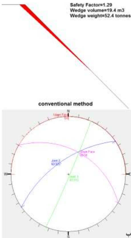
شکل ۹- اختلاف میان روش قطعی رایج و روش احتمالاتی شبیه سازی مونت کارلو در تعیین جهت داری ناپیوستگی ها و ریزش های سنگی. الف- روش احتمالاتی شبیه سازی مونت کارل؛ ب- روش قطعی رایج.
