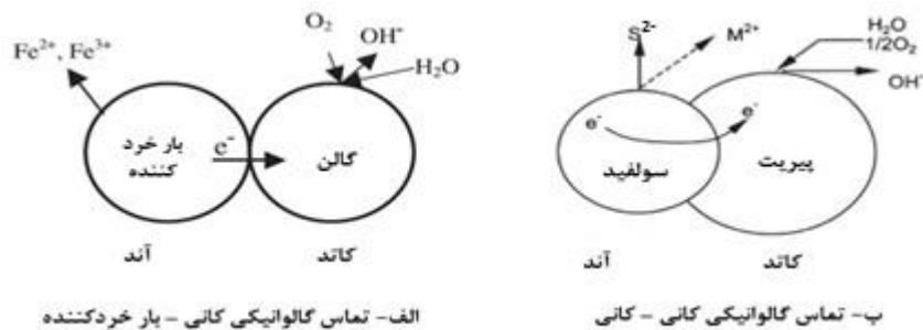
شکل ۱: مدل گالوانیکی حاصل از تماس بین کانی - کانی و کانی - بار خردکننده [۳]
