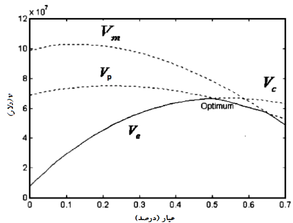
شکل ۳: منحنی‌های v_e ، v_p ، v_c و v_m [۱۸]
