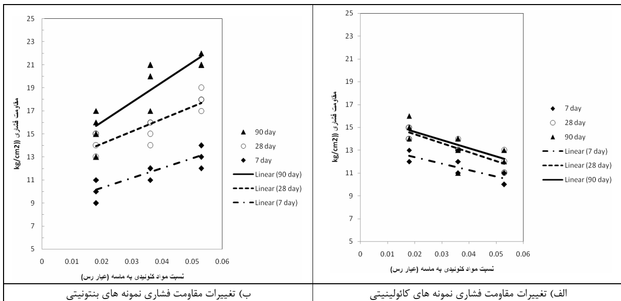
شکل ۲: تغییرات مقاومت فشاری نمونه‌ها
