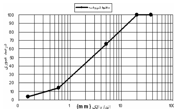
شکل ۱: منحنی دانه بندی
