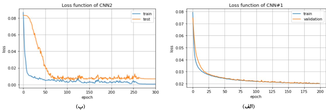
شکل ۶- نمودار الف- تابع هزینه شبکه CNN1، ب- CNN2
