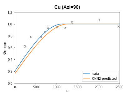
شکل ۱۳- مدل واریوگرام برازش شده به صورت دستی (خط آبی) و مدل CNN (خط نارنجی) برای سه عنصر مورد مطالعه منطقه نوچون
