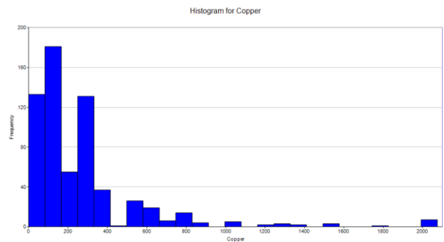
شکل ۱۰- هیستوگرام عنصر مس
