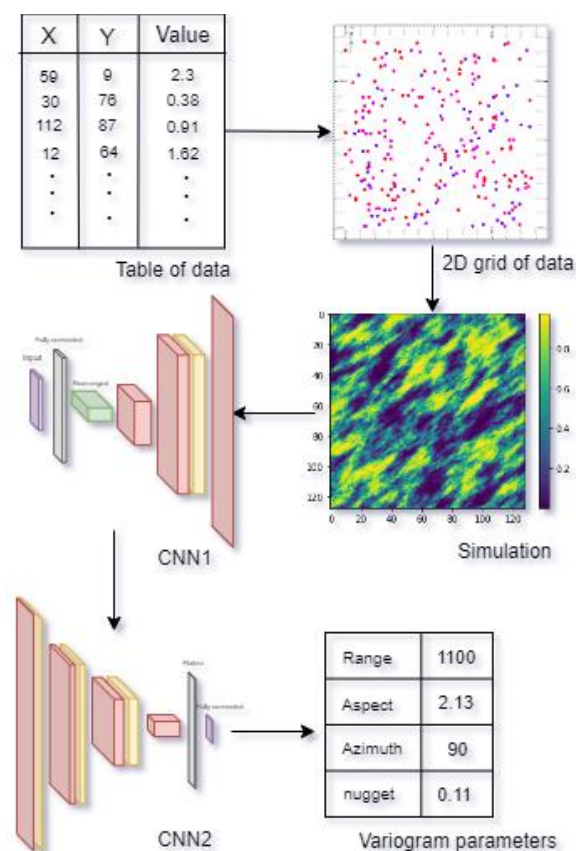
شکل ۲- فلوجارت کلی الگوریتم، با توجه به شکل داده‌های ورودی پس از شبیه‌سازی وارد شبکه CNN اول شده، خروجی شبکه CNN اول وارد شبکه CNN دوم می‌شود و پارامترها واریوگرام پیش‌بینی می‌شود
