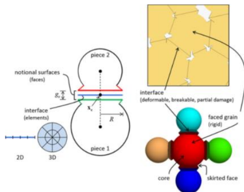
شکل ۴- نمایش شماتیک مدل اتصال تخت [۲۰]
