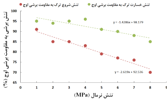
شکل ۱۳- تغییرات نسبت تنش شروع ترک و خسارت ترک به مقاومت برشی اوج برحسب تنش نرمال در آزمون‌های برش مستقیم عددی
