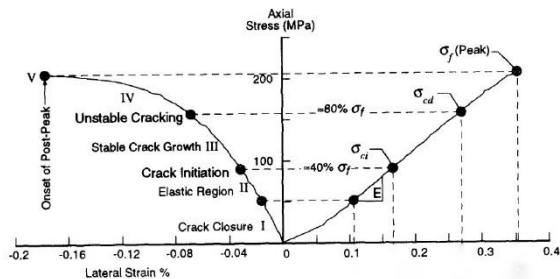
شکل ۲- دیاگرام تنش- کرنش محوری آزمون تک محوره فشاری بر روی گرانیت لاک دو بونت به همراه نمایش سطوح تنش مقاومت اوج، تنش شروع ترک و تنش خسارت ترک [۴]
