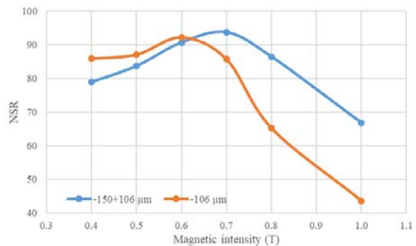
شکل ۹- تاثیر شدت میدان مغناطیسی بر آهنگ بازده کارخانه ذوب به دست آمده برای ذرات ۱۵۰-۱۰۶+ و ۱۰۶- میکرون.
