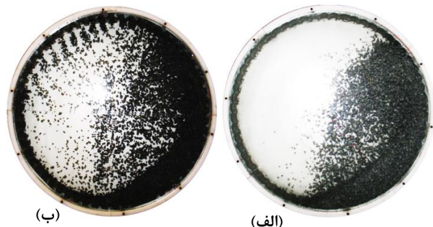
شکل ۲۱- الف) آستر ساییده شده و ب) آستر نو سرچشمه در سرعت ۸۵ درصد و پرشدگی ۱۵ درصد
