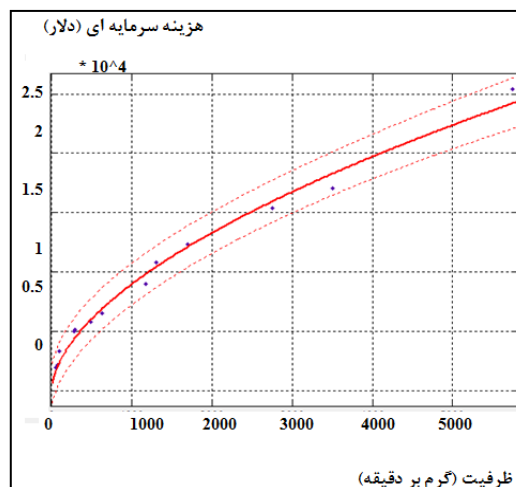
شکل ۴. روند تغییرات هزینه هیدروسیکلون استاندارد
