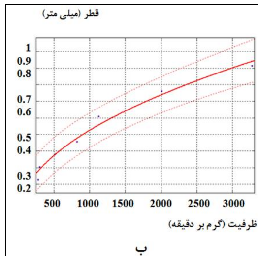
شکل ۶. نمودار رابطه بین قطر و ظرفیت دو نوع هیدروسیکلون
