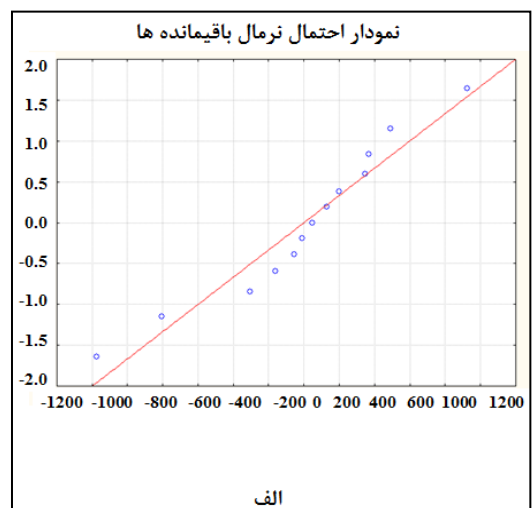
شکل ۸. هیستوگرام باقیمانده‌ها و نمودار احتمال نرمال برای مدل‌های چند متغیره هزینه سرمایه‌ای هیدروسیکلون استاندارد
