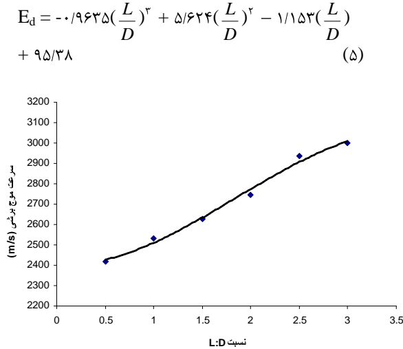
شکل ۵: ارتباط سرعت موج برشی و نسبت طول به قطر نمونه.
